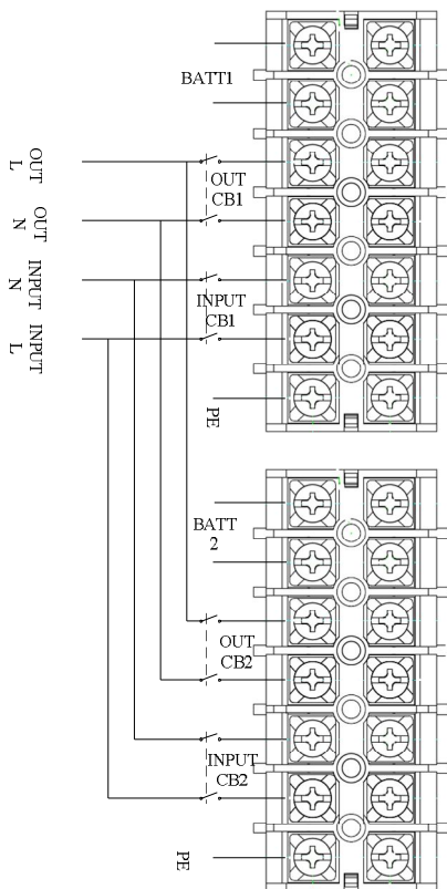
Рис. 2-6. Схема параллельной проводки
