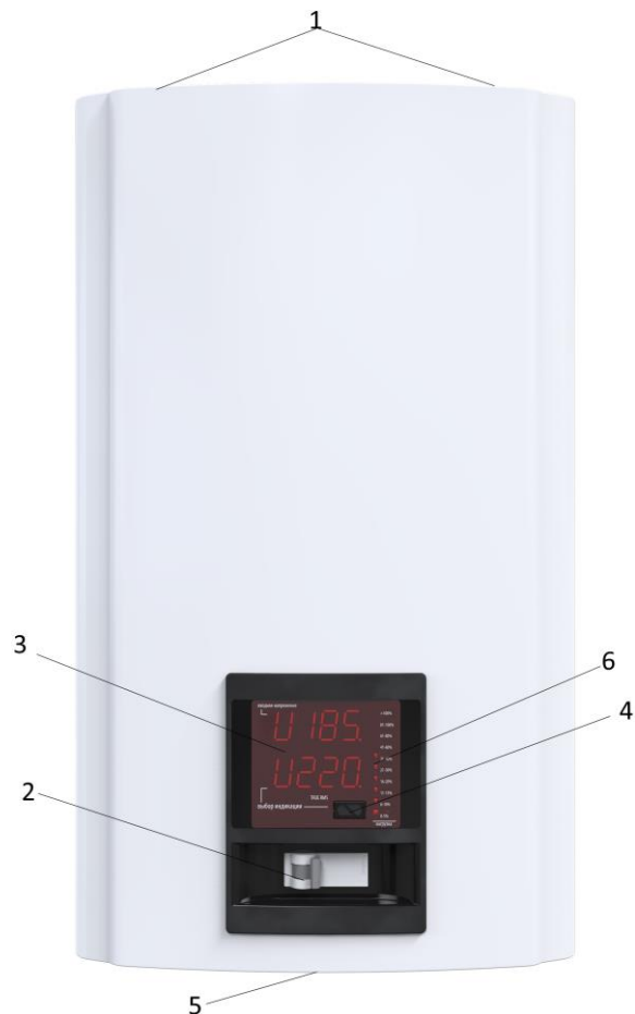
Рис.3 Внешний вид стабилизатора Герц-Дуо У 16-1/XXX V3.0
