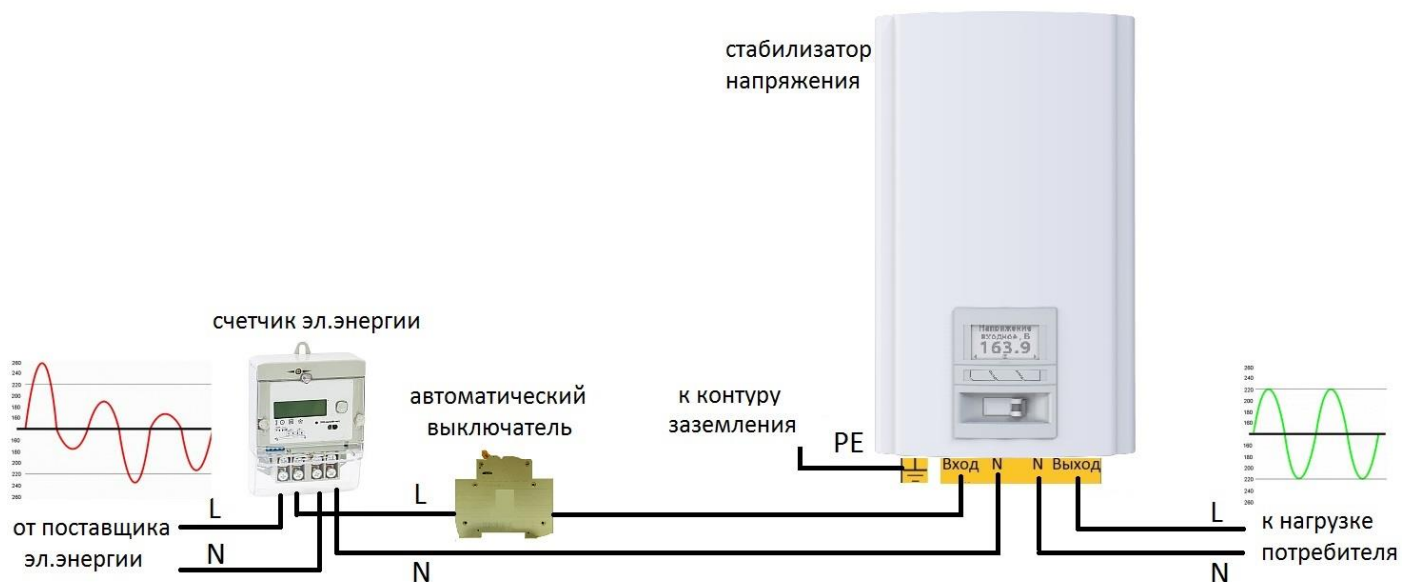
Рисунок 11. Схема подключения Герц и Герц-Дуо к однофазной сети
