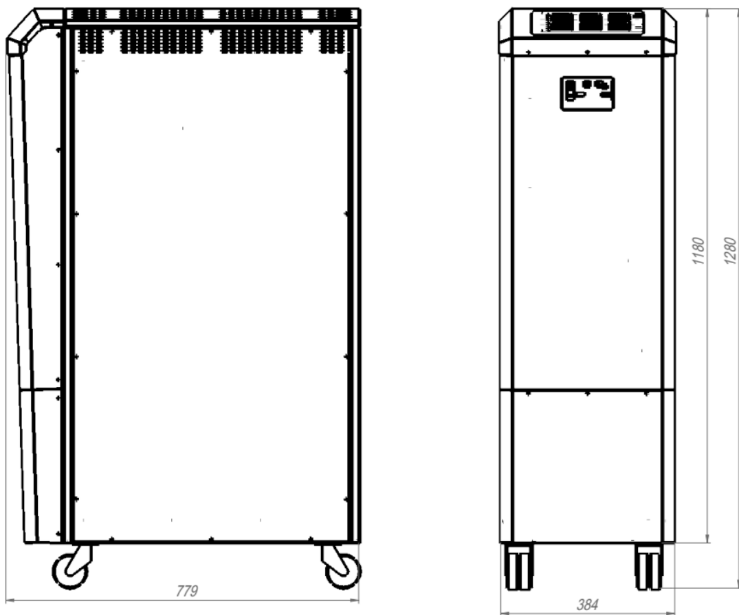
Рисунок 9. Габаритні розміри стабілізатора Герц-ПРО на 100-160А
