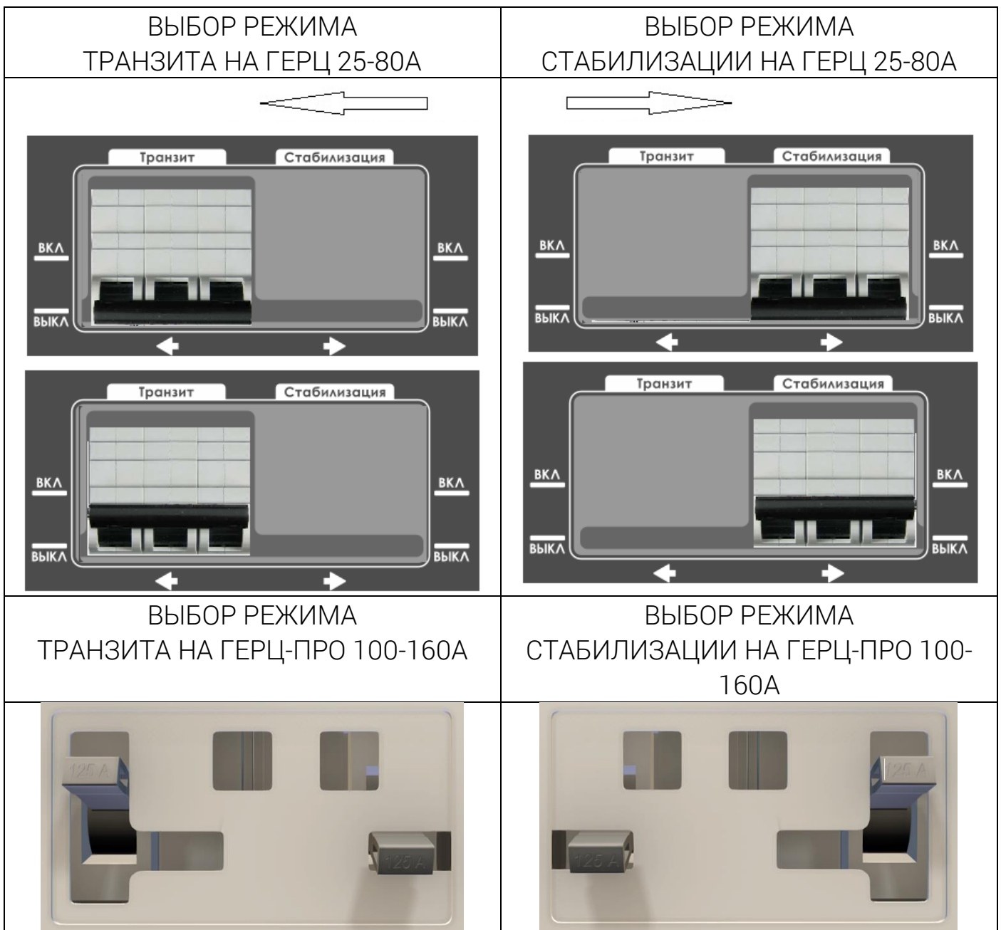
Рисунок 13. Порядок переключения между режимами работы стабилизатора
