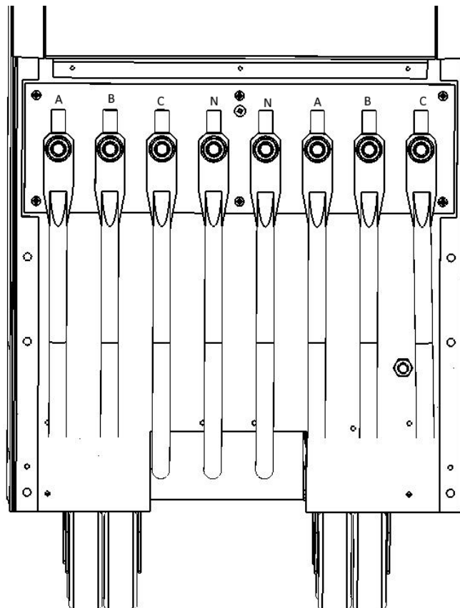
Рисунок 6. Внешний вид передней части стабилизатора Герц-ПРО на 100-160А
