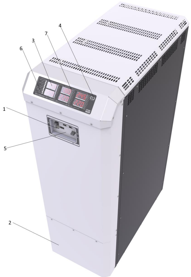
Рисунок.4 Зовнішній вигляд стабілізатора Герц-ПРО на 100-160А
