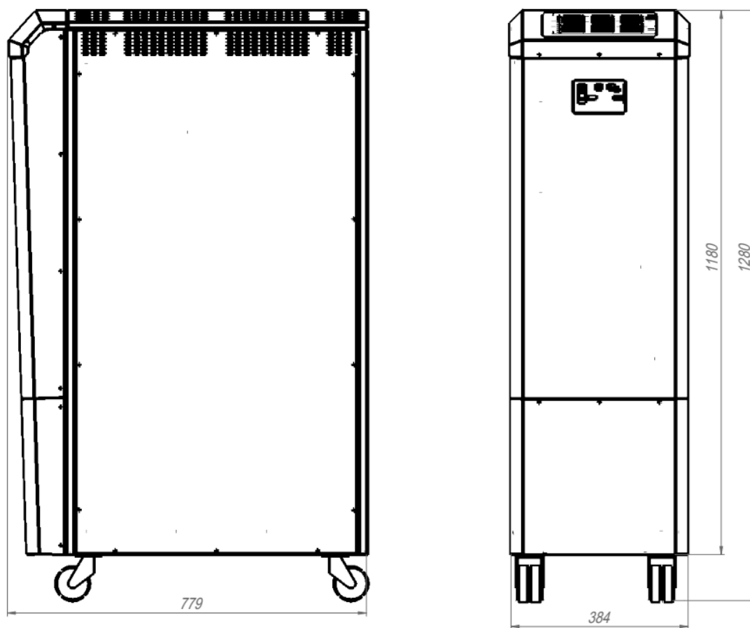
Рисунок 9. Габаритные размеры стабилизаторов Герц-ПРО на 100-160А
