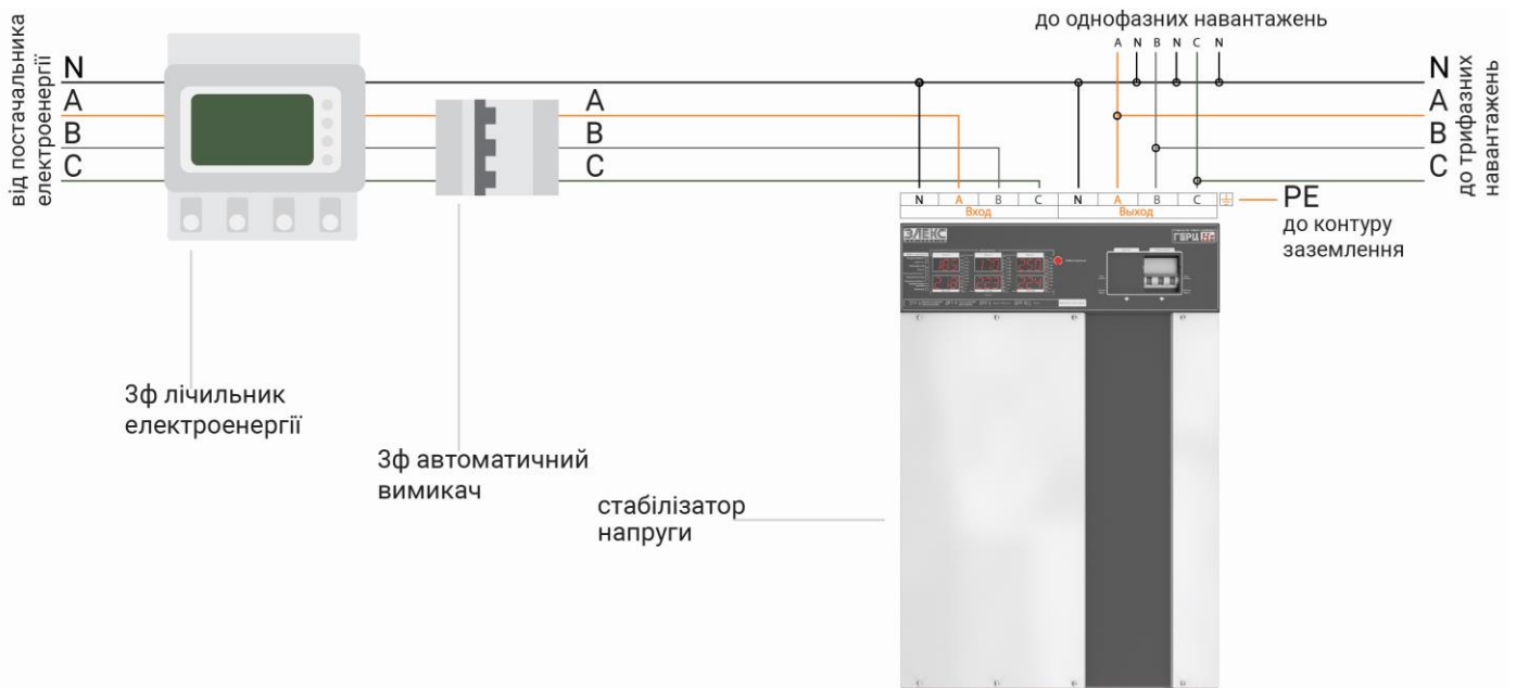
Рисунок 10. Схема підключення стабілізатора до трифазної мережі
