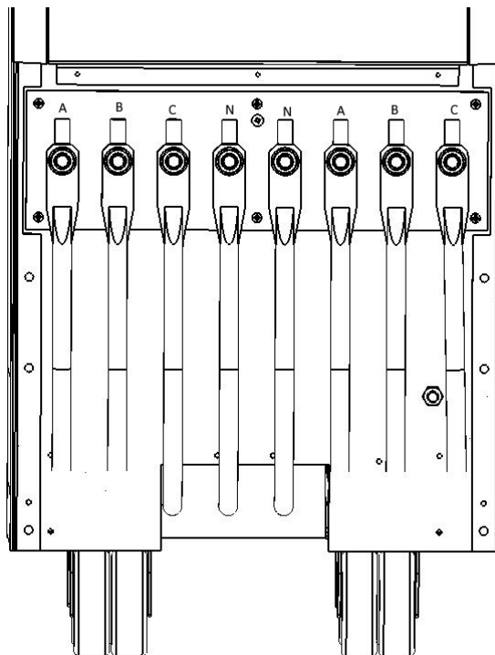
Рисунок 6. Зовнішній вигляд передньої частини стабілізатора Герц-ПРО на 100-160А без кришки
