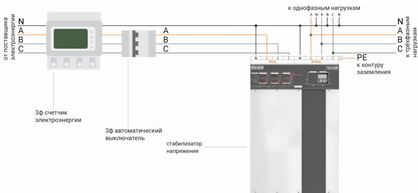
Рисунок 10. Схема подключения стабилизатора к трёхфазной сети
